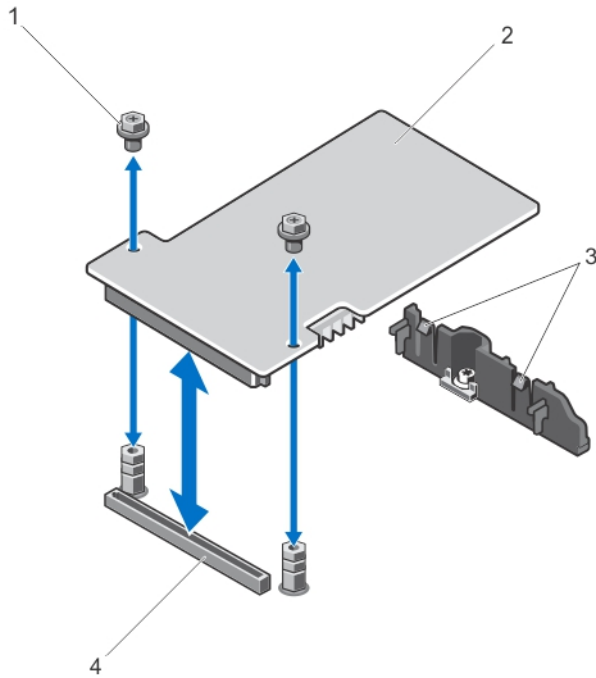
그림 24. 저장소 컨트롤러 카드 분리 및 설치
