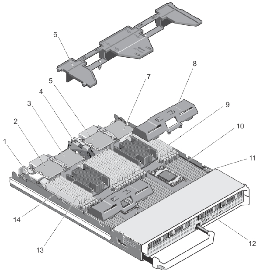
그림 5. 블레이드 내부
