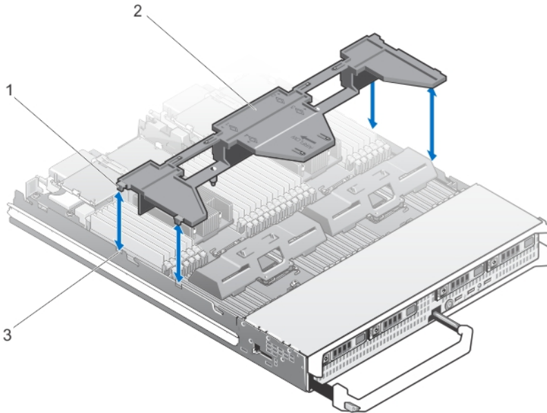
그림 6. 냉각 덮개 분리 및 설치
