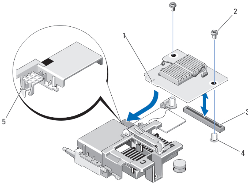
그림 12. 네트워크 도터 카드/LOM 라이저 카드 분리 또는 설치
