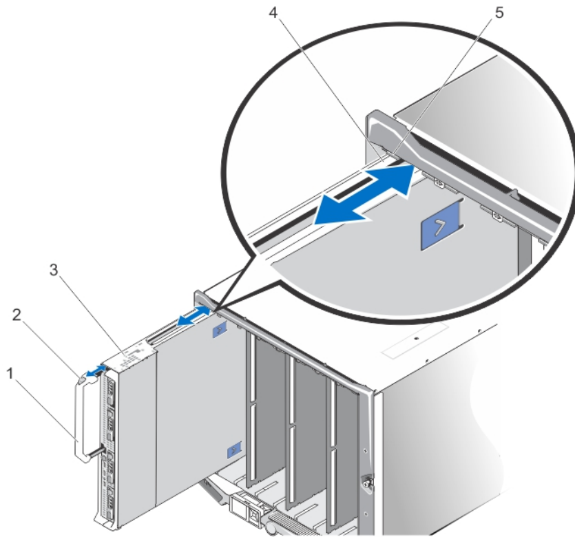
그림 3. 블레이드 분리 및 설치
