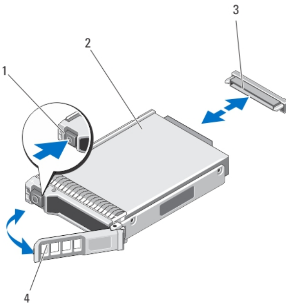
그림 7. 하드 드라이브/PCIe SSD 분리 및 설치
