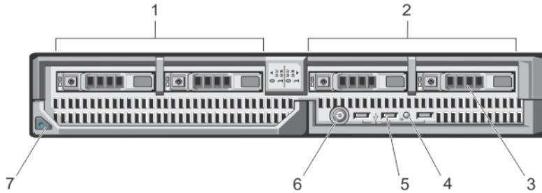
그림 1. 전면 패널 구조 및 표시등
