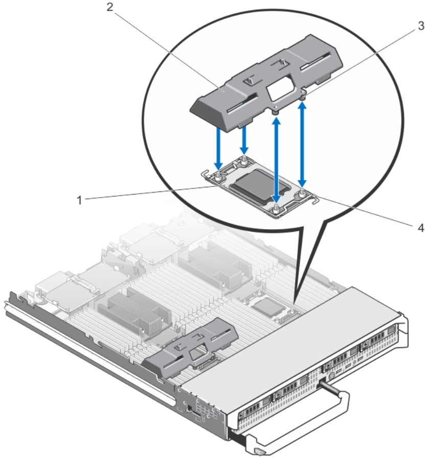
그림 16. 프로세서/DIMM 보호물 분리 및 설치
