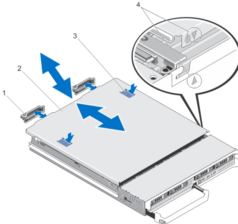
그림 4. 블레이드 열기 및 닫기
