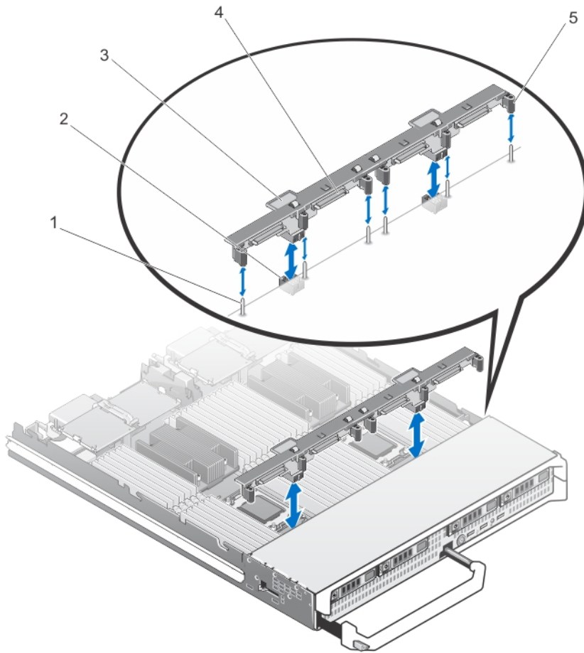
그림 9 . Hard-Drive/SSD 후면판 분리 및 설치(전체 길이)
