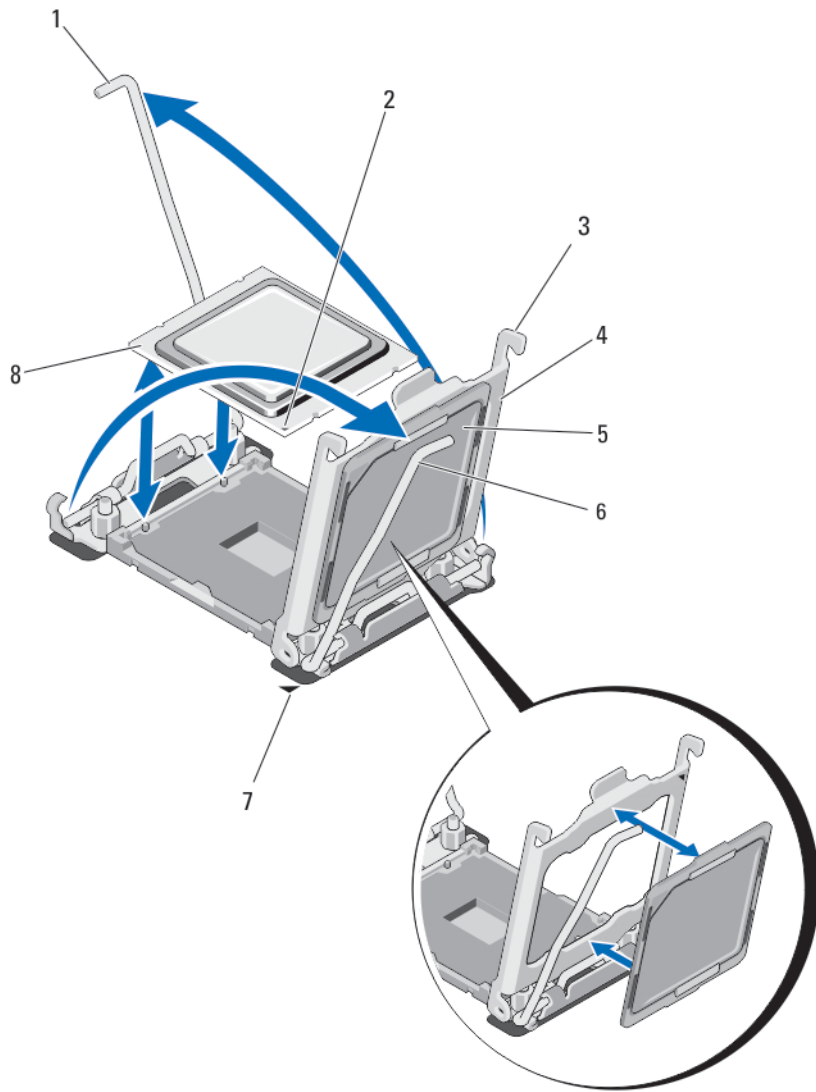
그림 19. 프로세서 분리 및 설치
