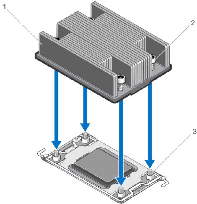
그림 17. 방열판 분리 및 설치
