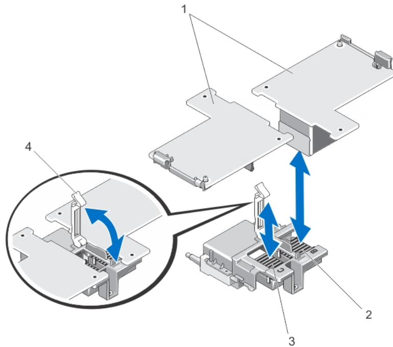
그림 11. 메자닌 카드 분리 및 설치
