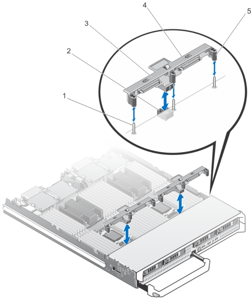
그림 10 . Hard-Drive/SSD 후면판 분리 및 설치(절반 길이)
