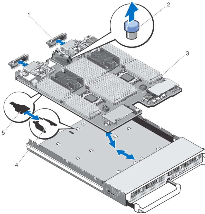
그림 20. 시스템 보드 분리 및 설치
