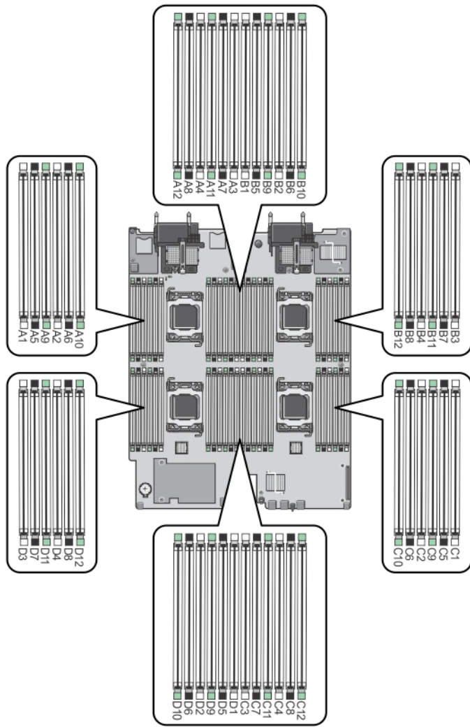
그림 21. 메모리 소켓 위치
