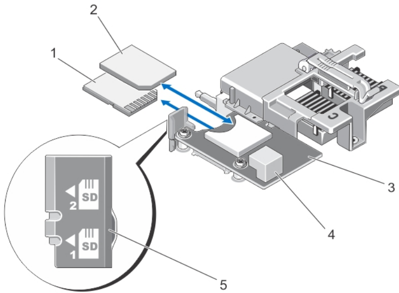
그림 13. SD 카드 장착
