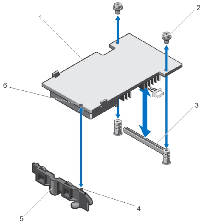
그림 25. PCIe 확장기 카드 분리 및 설치
